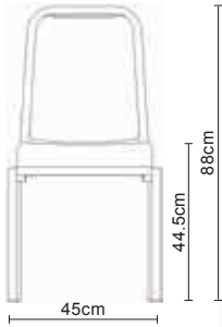
60/1 Depth 57cm Weight 5.2kg
