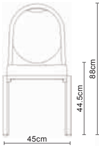
60/2 Depth 57cm Weight 5kg
